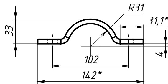
Поз.4 (Полухомут)
